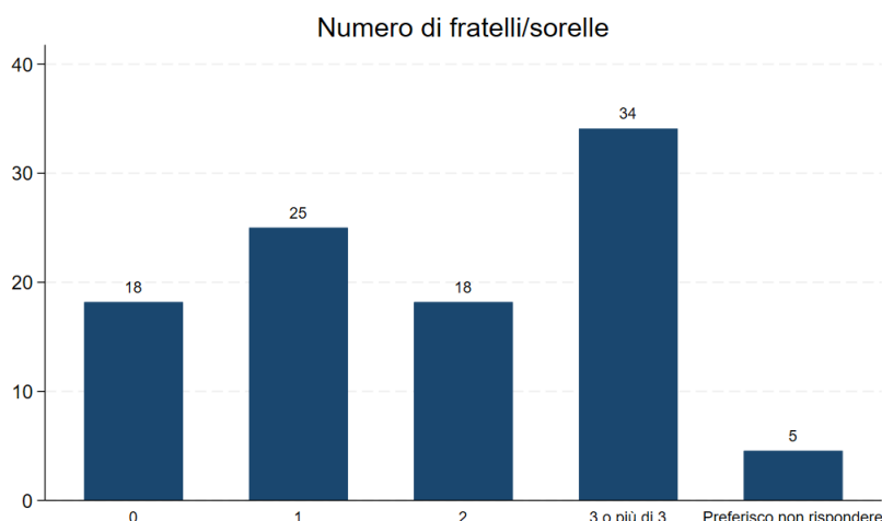
Figura 4: Numerosità famiglia
